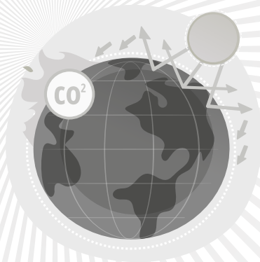
אפקט החממה
